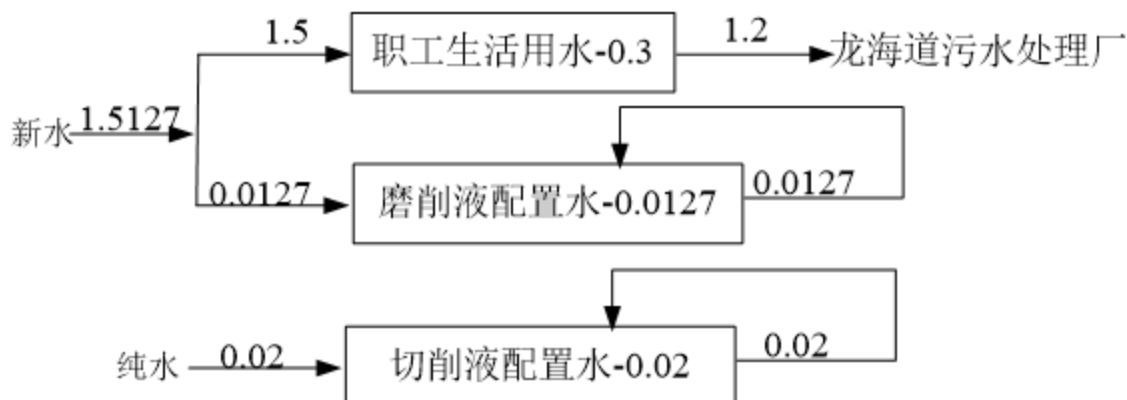
图 5 本项目建成后全厂水平衡图 \text{m}^3/\text{d}
