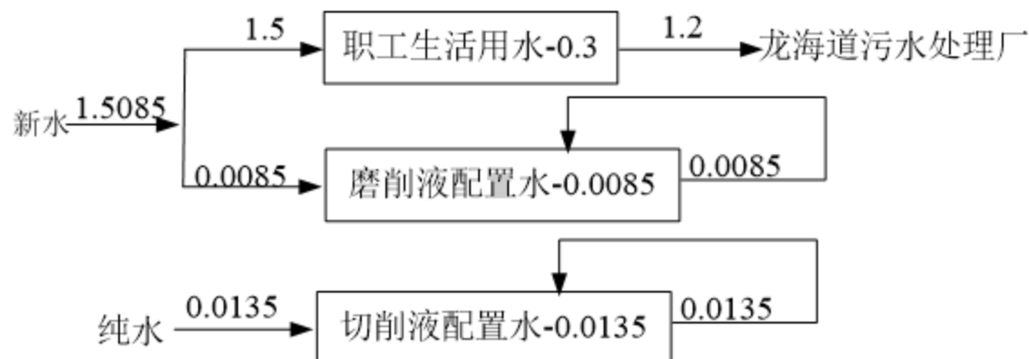
图 2 现有工程水平衡图 \text{m}^3/\text{d}
