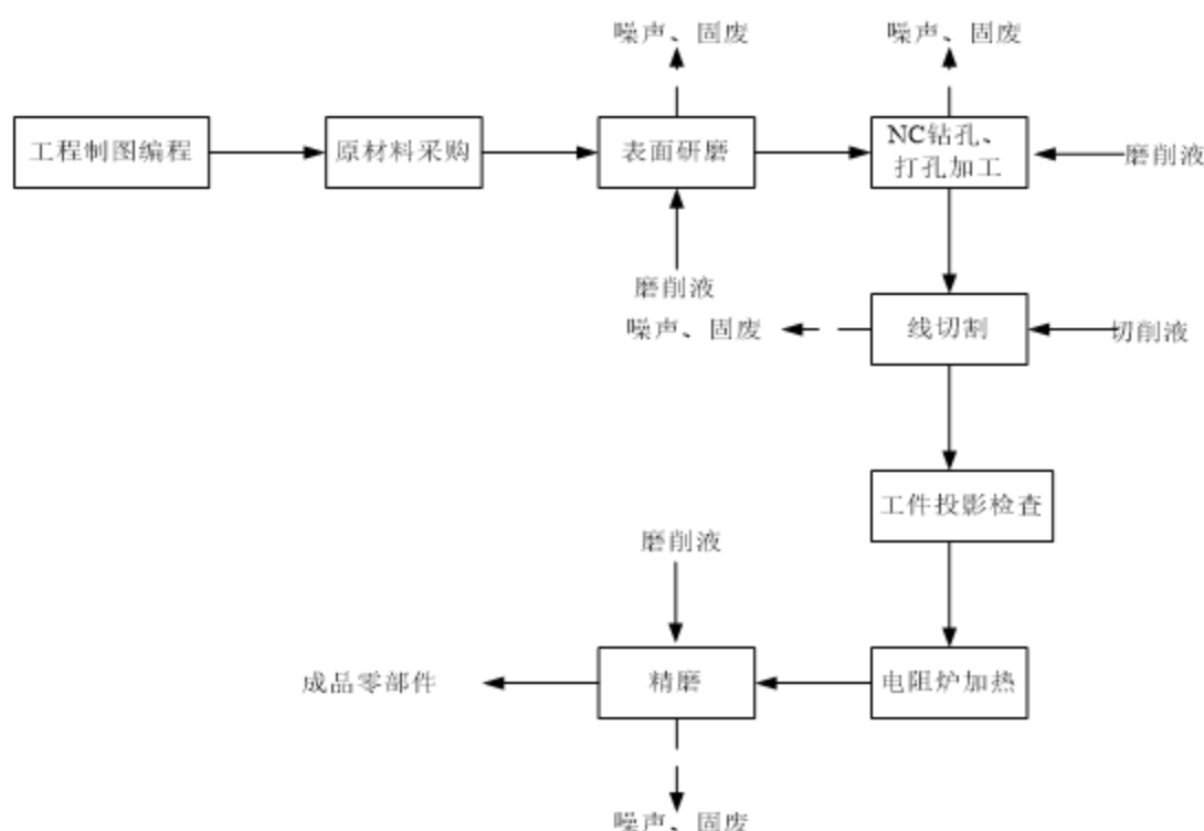
图 6 本项目生产工艺流程图
